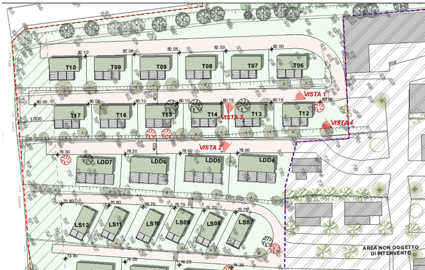
Planimetria individuazione viste RENDER
