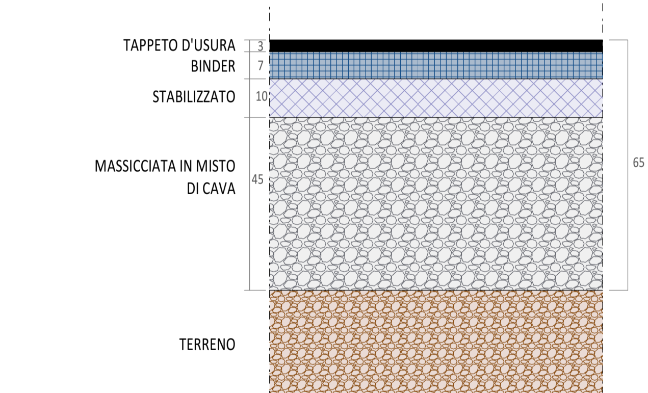
SEZIONE STRADA tratto B - scala 1:10
