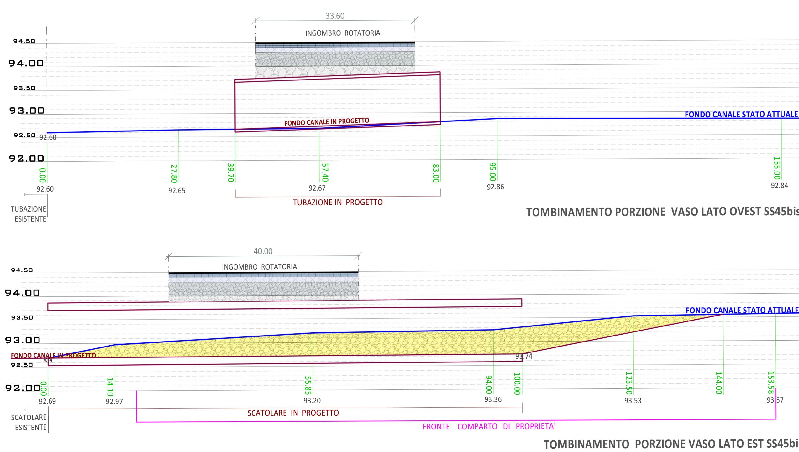
TOMBINAMENTO PORZIONE VASO LATO EST SS45BIS
