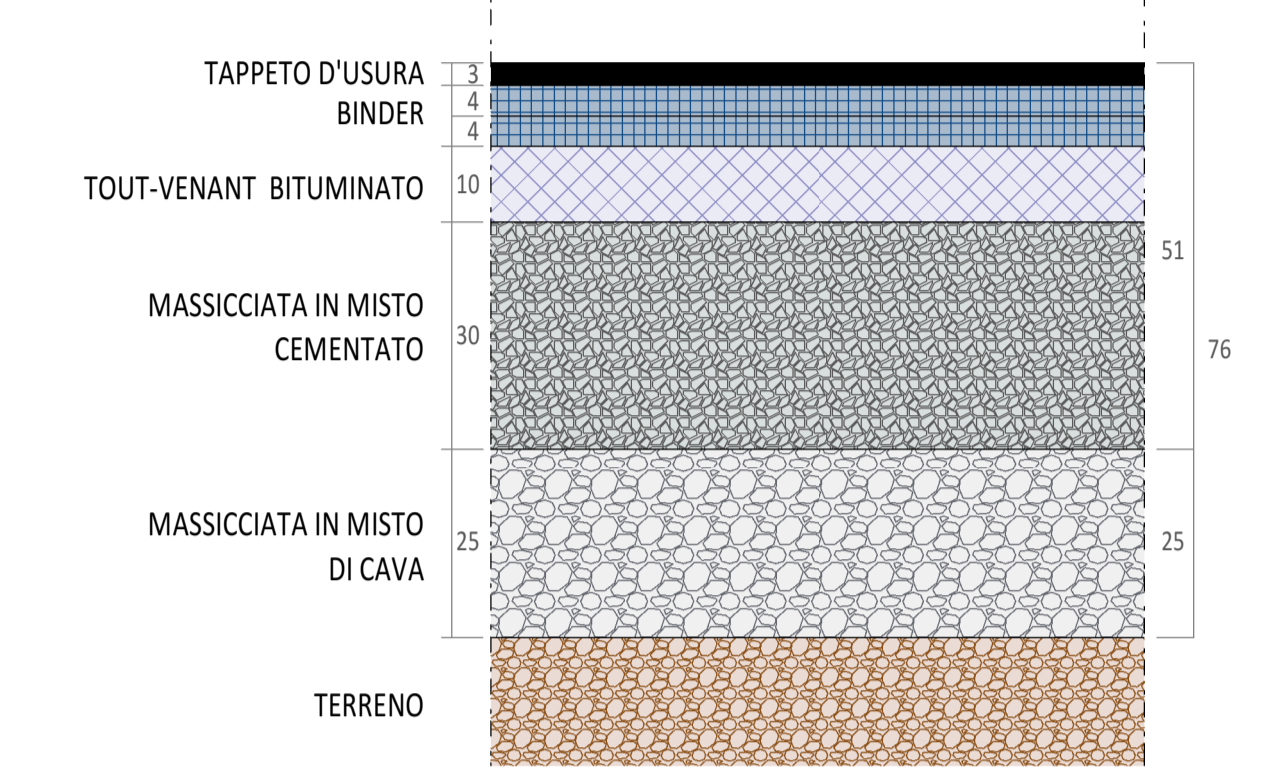
SEZIONE STRADA tratto A - scala 1:10
