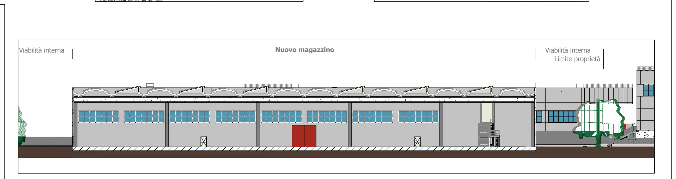
PIANTA SEZIONE-VISTA - SCALA 1 : 400
