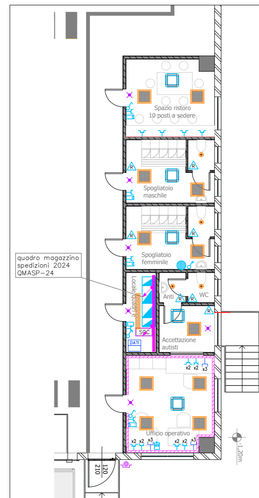
LOCALI DI SERVIZIO - SCALA 1 : 100
