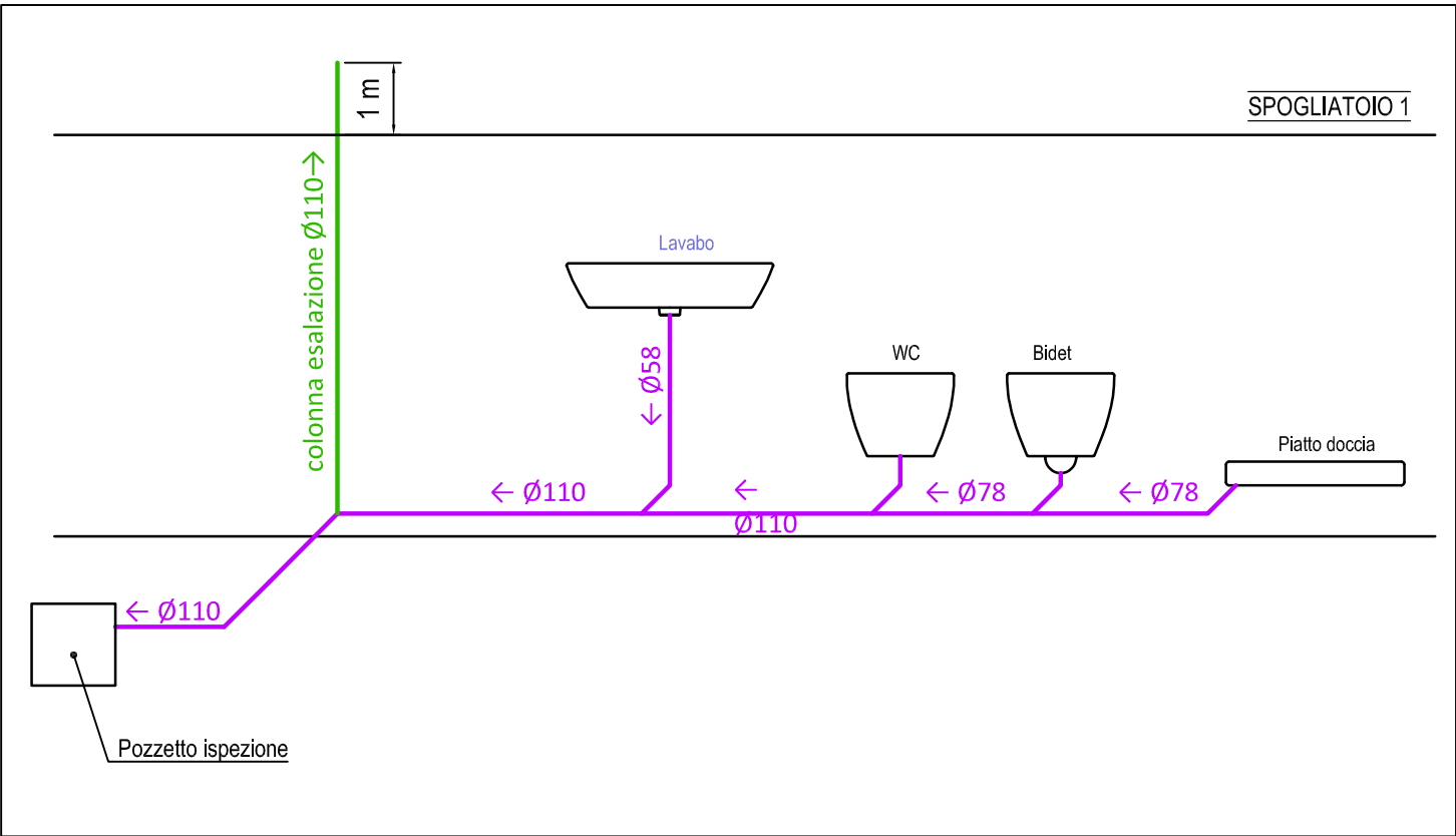
SCHEMA ALTIMETRICO TIPICO
